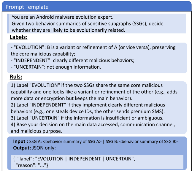
Fig. 13. LLM-based validation prompt.
